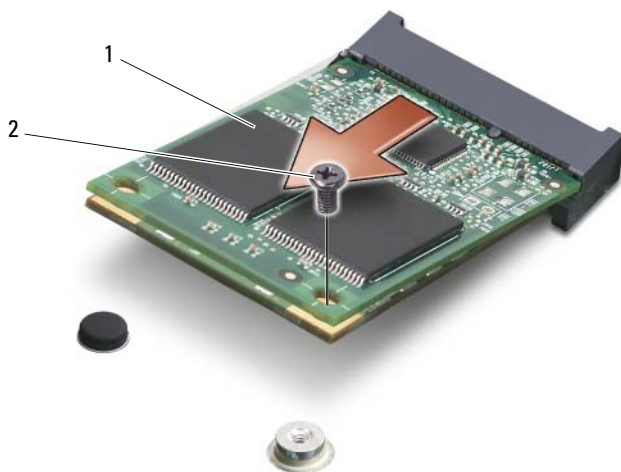
1 FCM 卡 2 M2 x 3 mm 固定螺絲
